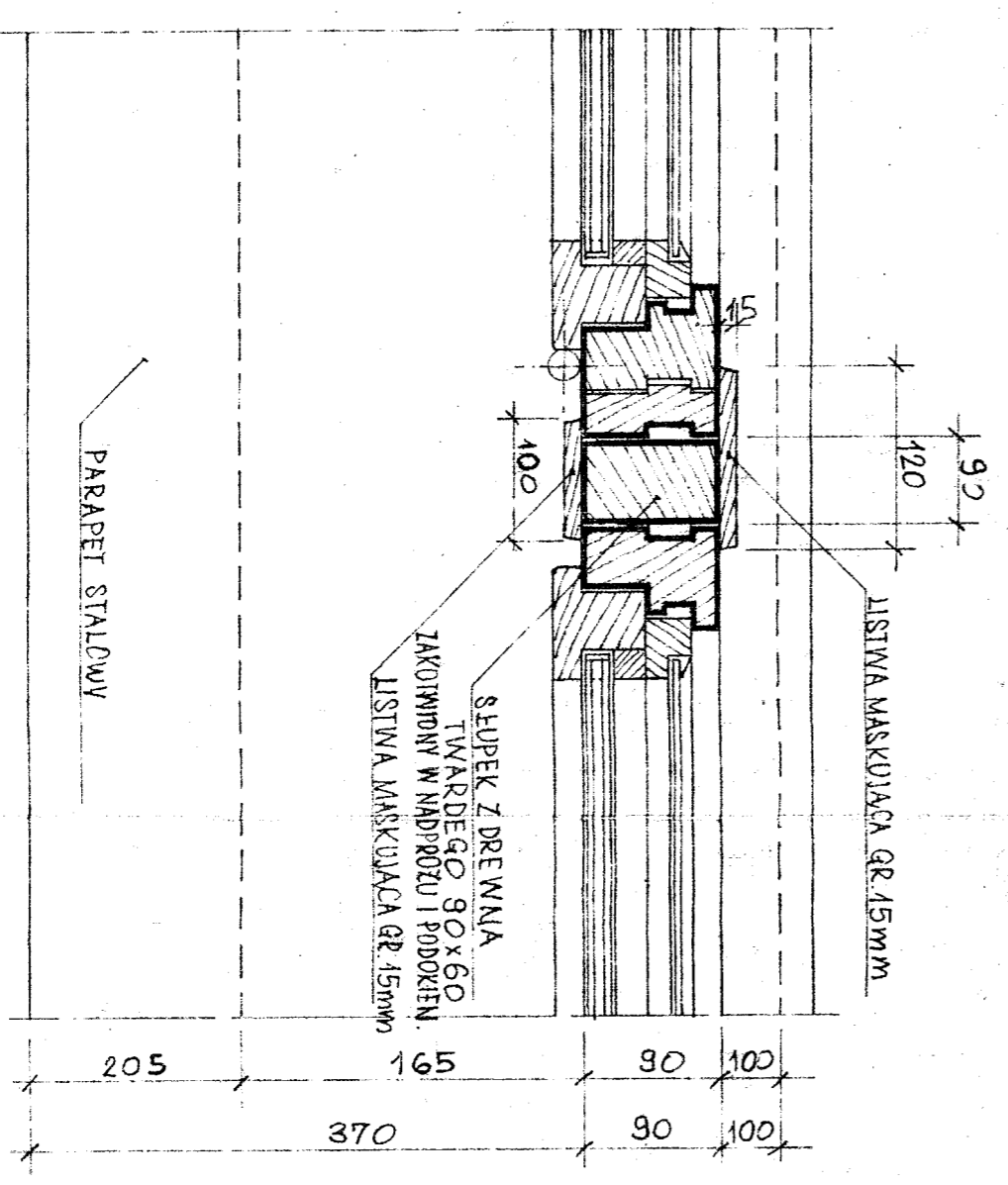
OKNA ZESPOLONE ZE ŚLUPKIEM DREWNIANYM SZER 60mm
